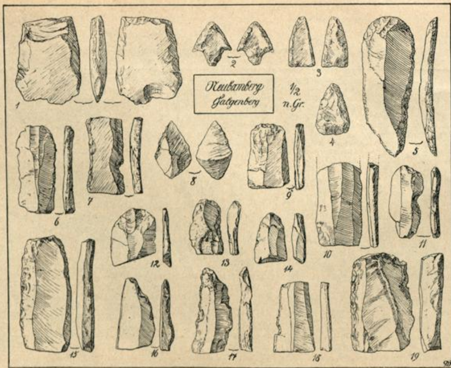
Abb. 3. Neolithische Feuersteingeräte
