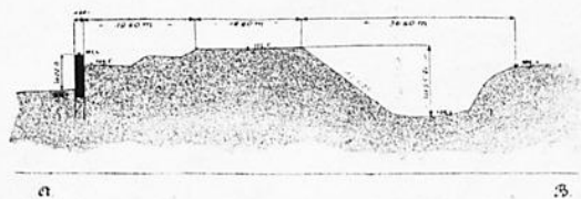
Schnitt A-B
