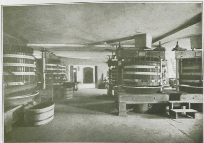
Modernes Kelterhaus mit hydraulischen Weinpressen
